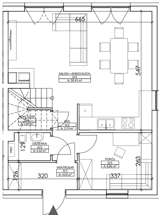
RZUT PARTERU
