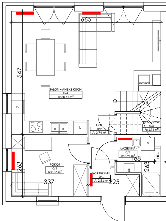
RZUT PARTERU
