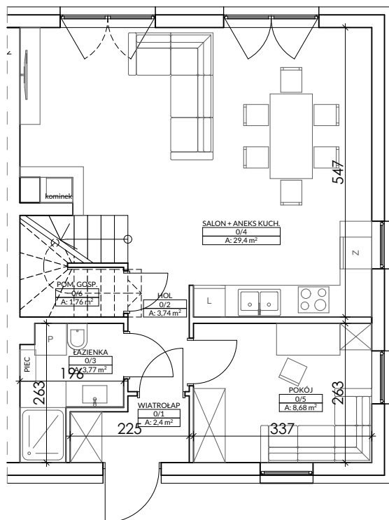
RZUT PARTERU ▲
